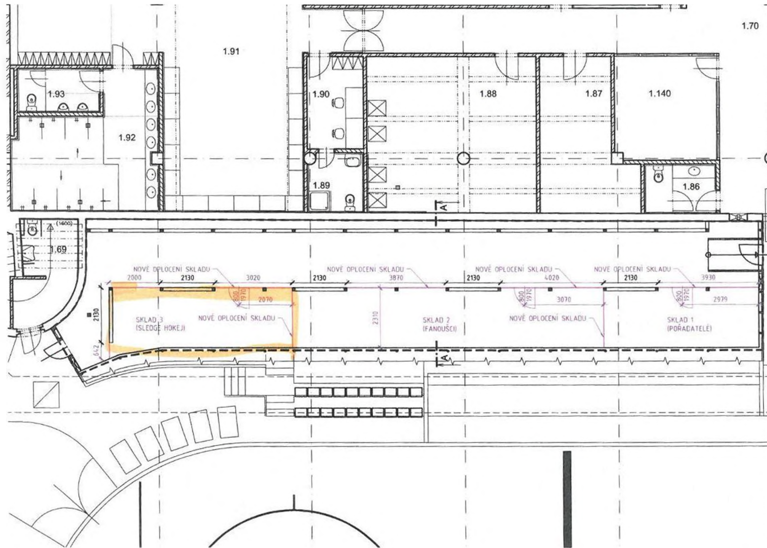
Zimní stadion České Budějovice - stavební úpravy - prostor pod západní tribunou I. LP NOVÉ OPLOCENÍ JEDNOTLIVÝCH SKLADŮ (pořadatelé, fanoušci, sladge hokej)
