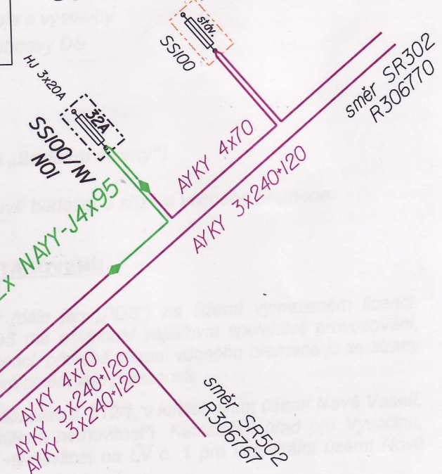
Schéma zapojení sítě NN
