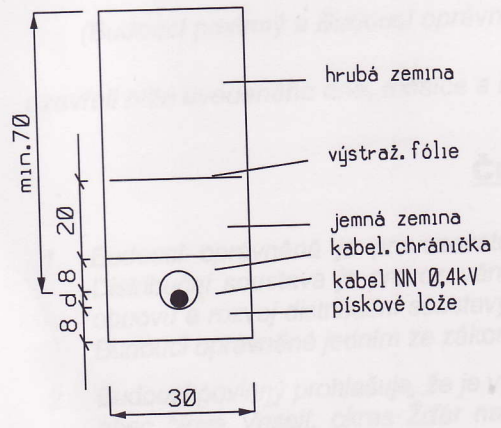
Řez uložení kabelu v zemi
