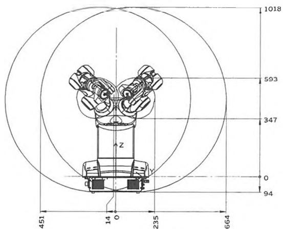
IRB 14000-0.5/0.5 Pohled zepředu
