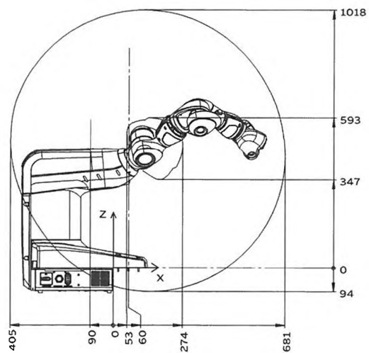
IRB 14000-0.5/0.5 Pohled z boku
