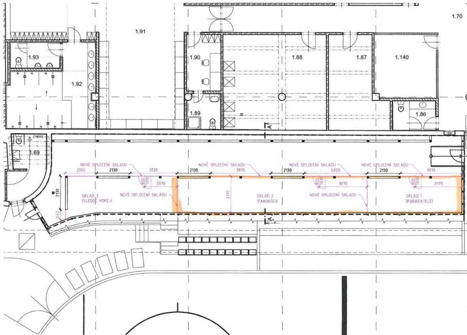
Zimní stadion České Budějovice - stavební úpravy - prostor pod západní tribunou I. LP NOVÉ OPLOCENÍ JEDNOTLIVÝCH SKLADŮ (pořadatelé, fanoušci, sladce hokej)
