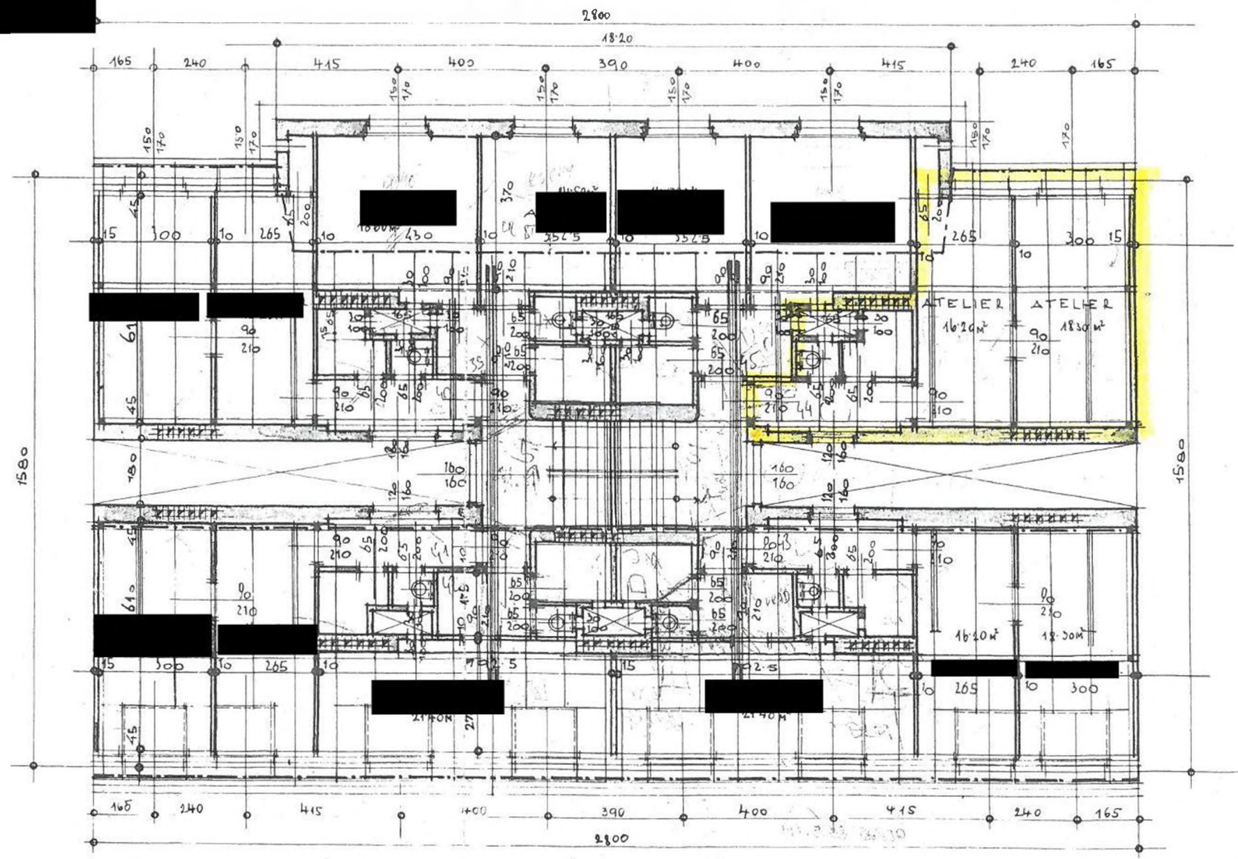
PODKROVÍ A KROV. 1:100.
