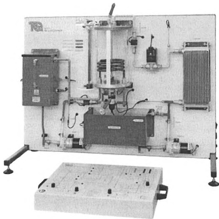
Trenažér procesů TecQuiment CE117 včetně experimentálního modulu
