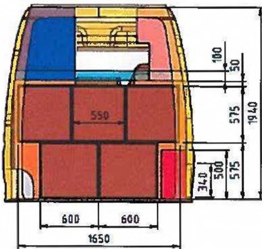
Mercedes Sprinter - sedák složený M 1:30 A3
