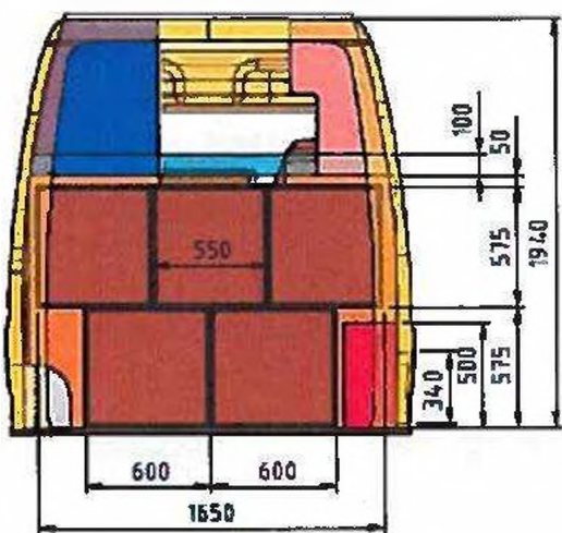
Mercedes Sprinter - sedák rozložený M 1:30 A3
