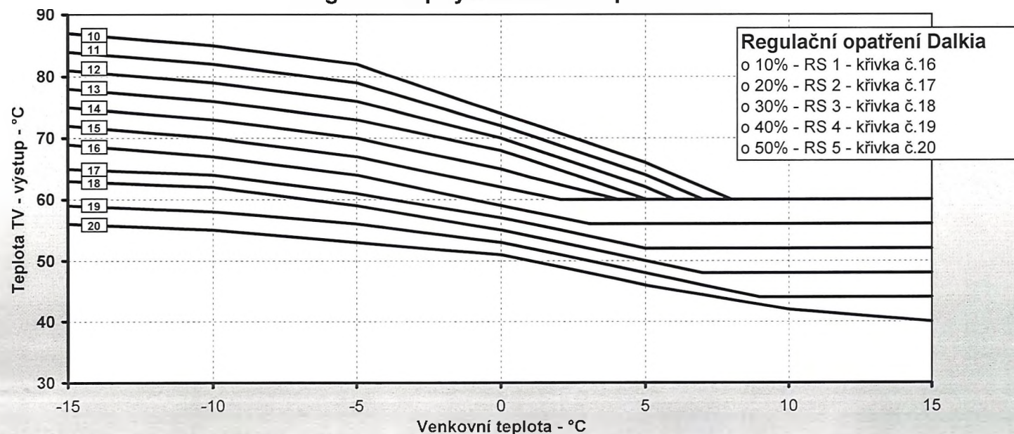
Diagram otopných křivek - topná voda
