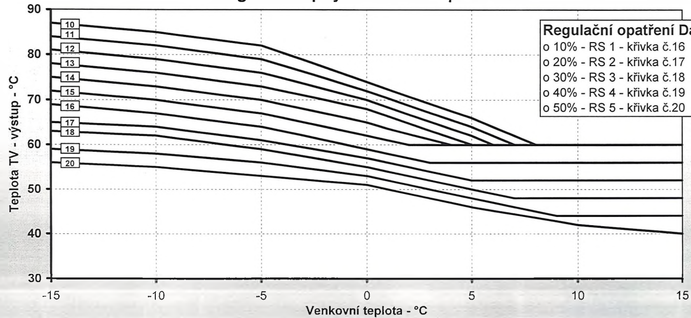
Diagram otopných křivek - topná voda
