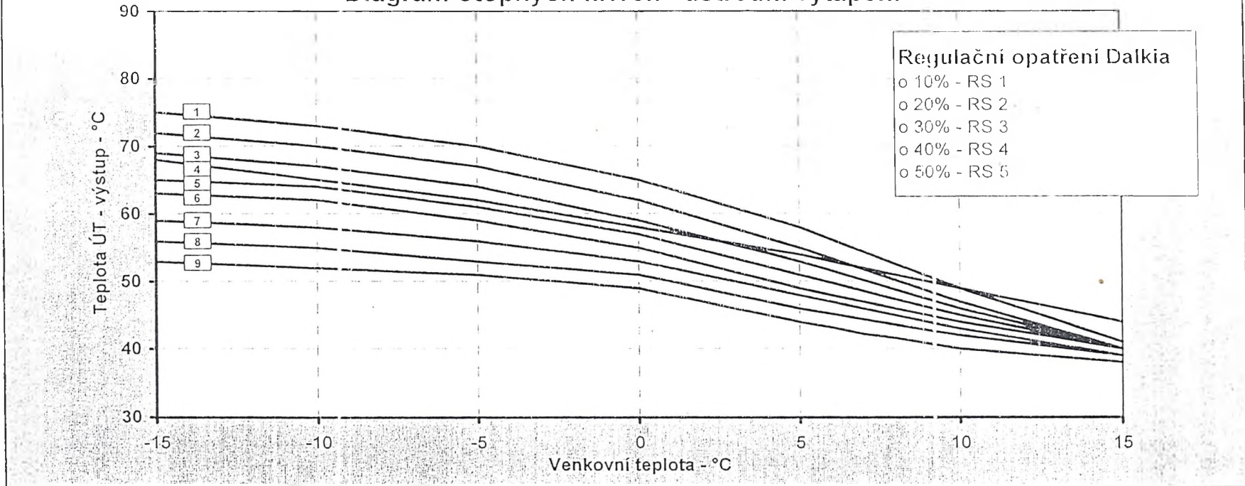
Diagram otopných křivek - ústřední vytápění
