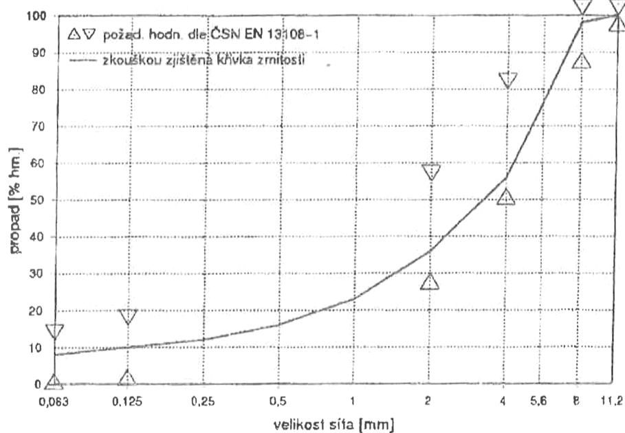
křivka zrnitosti ACO B 50/70
