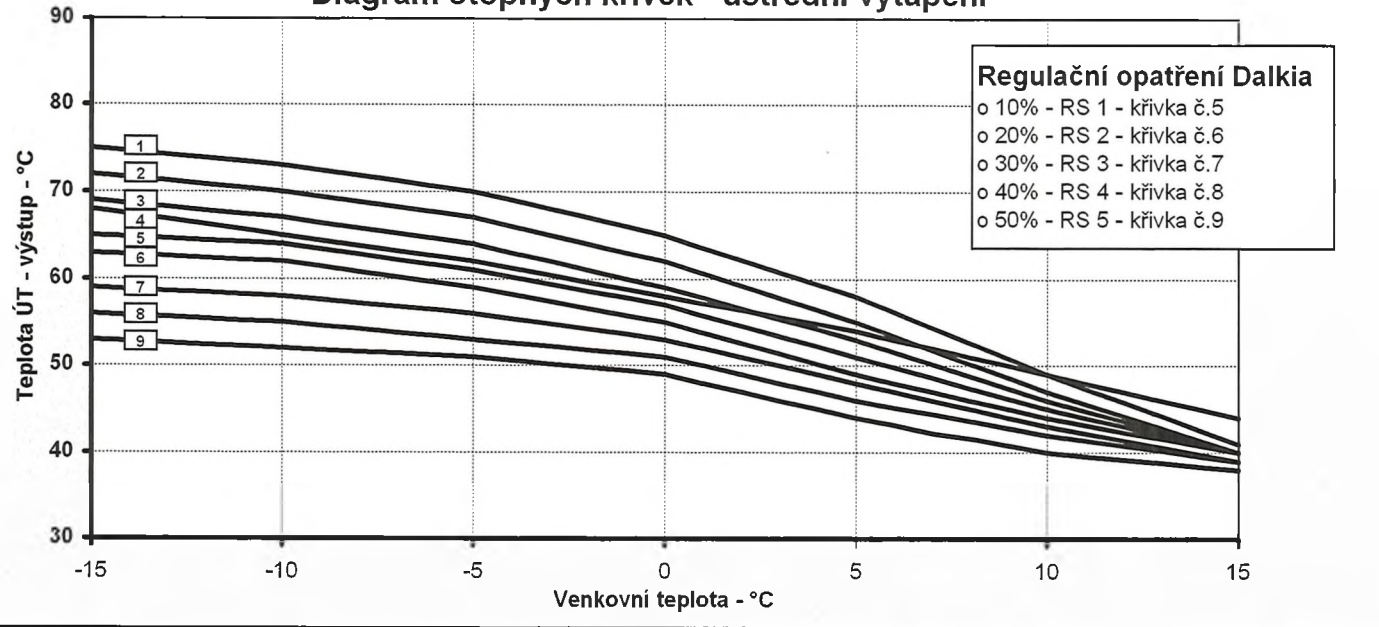
Diagram otopných křivek - ústřední vytápění
