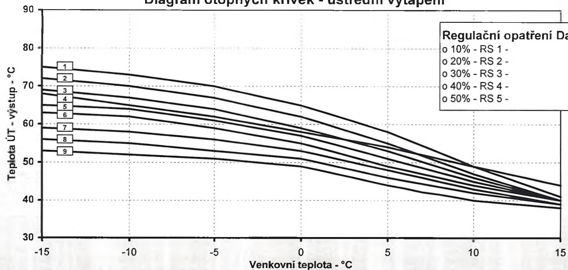
Diagram otopných křivek - ústřední vytápění
