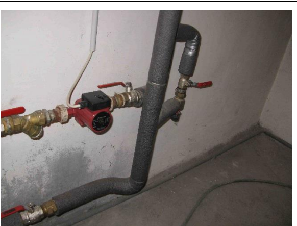
Potrubní systémy a oběhové čerpadlo Grundfos RS 25/4 G
