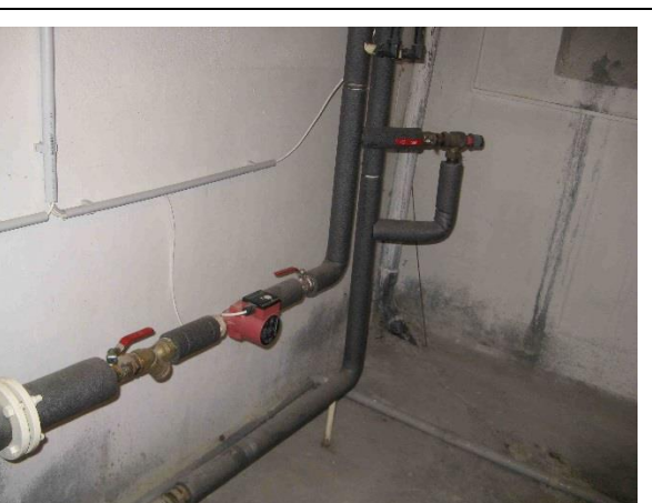
Potrubní systémy a oběhové čerpadlo Grundfos UPS 25-40
