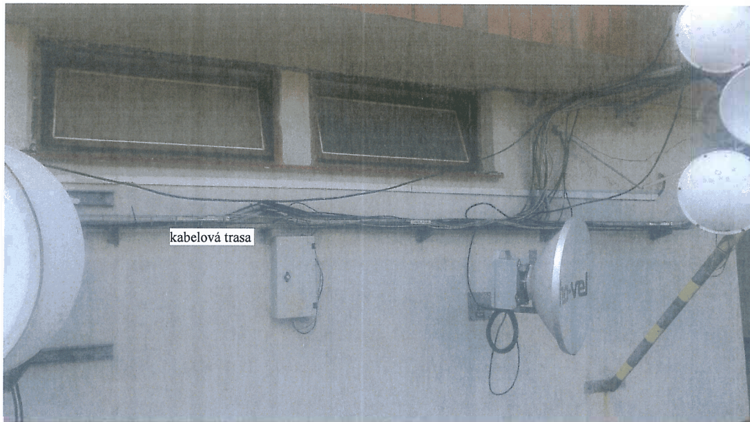
Obr. č.4, Kabelová trasa ve stávajících kabelových roštích
