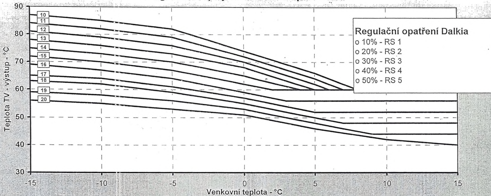
Diagram otopných křivek - topná voda
