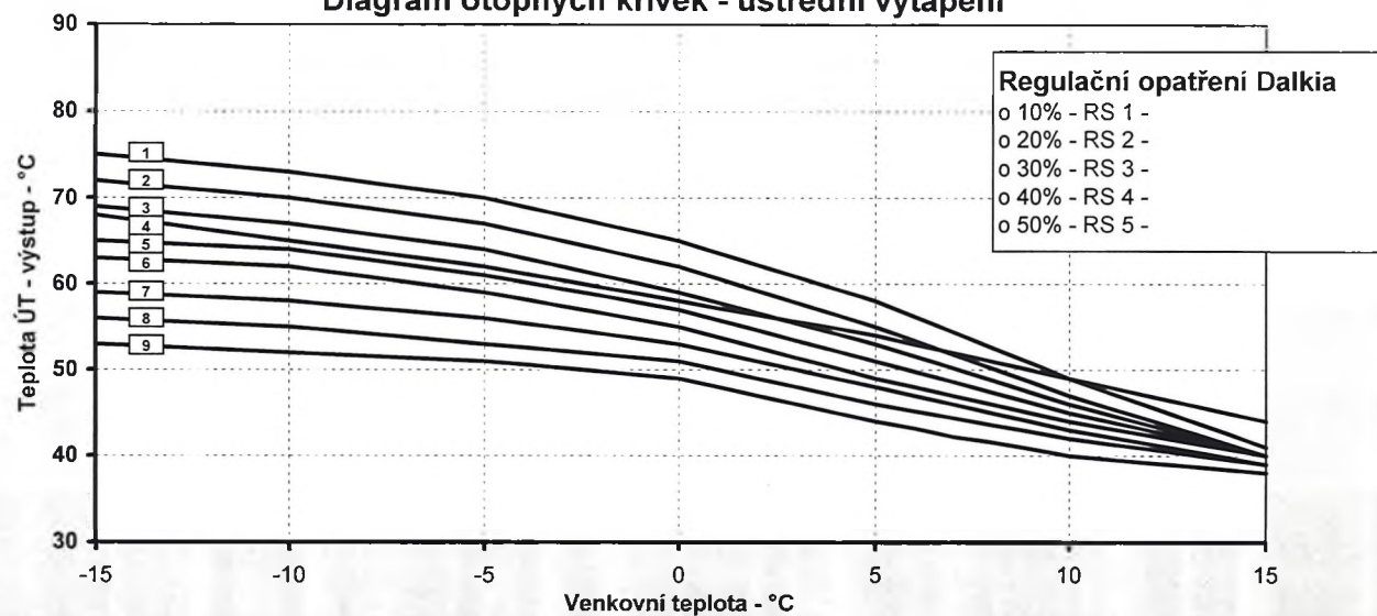
Diagram otopných křivek - ústřední vytápění
