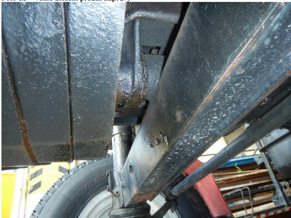
Foto č.5 – volné uložení přední nápravy
