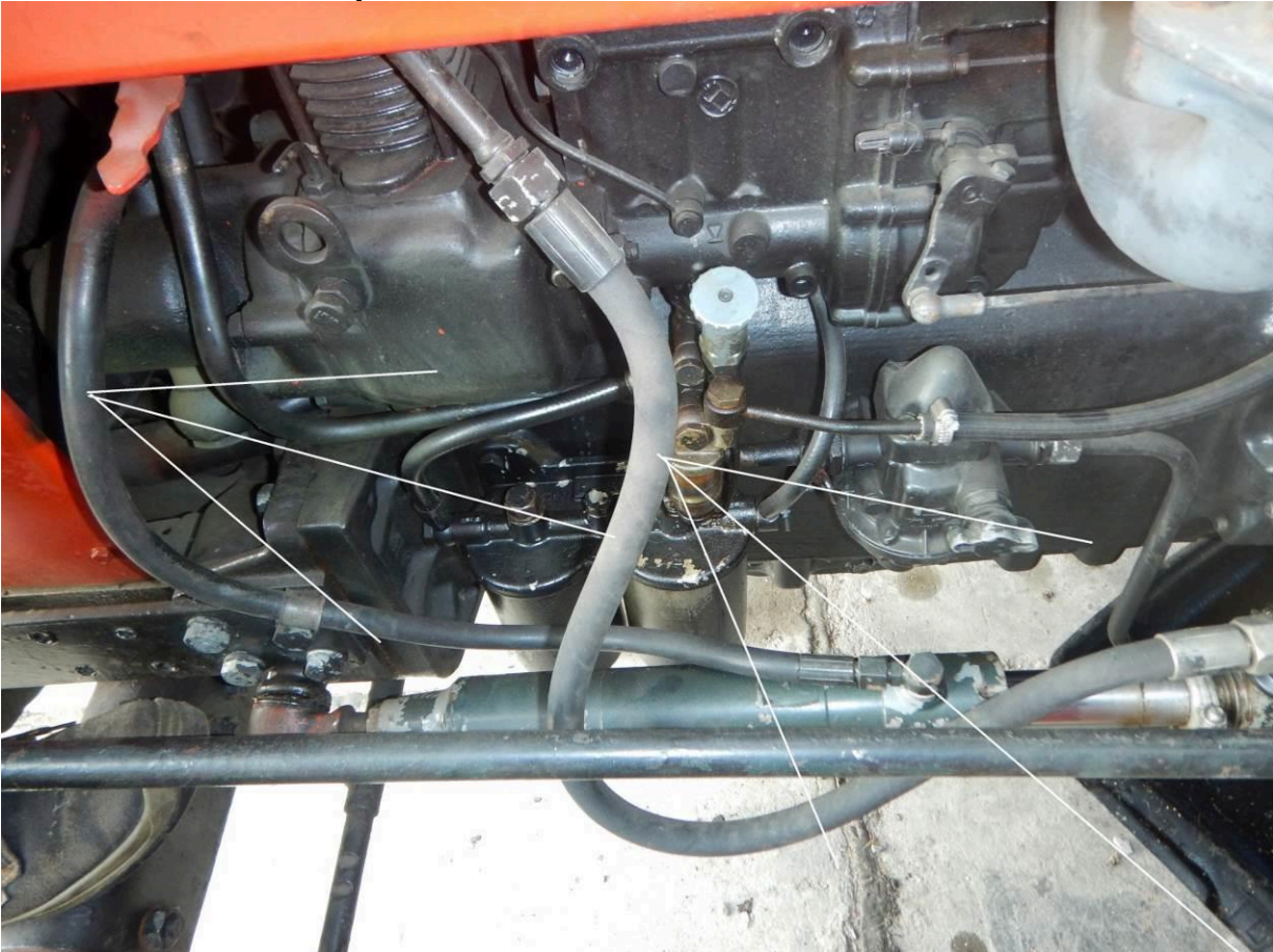
Foto č.3 – zteřelé hadice posilovače řízení
