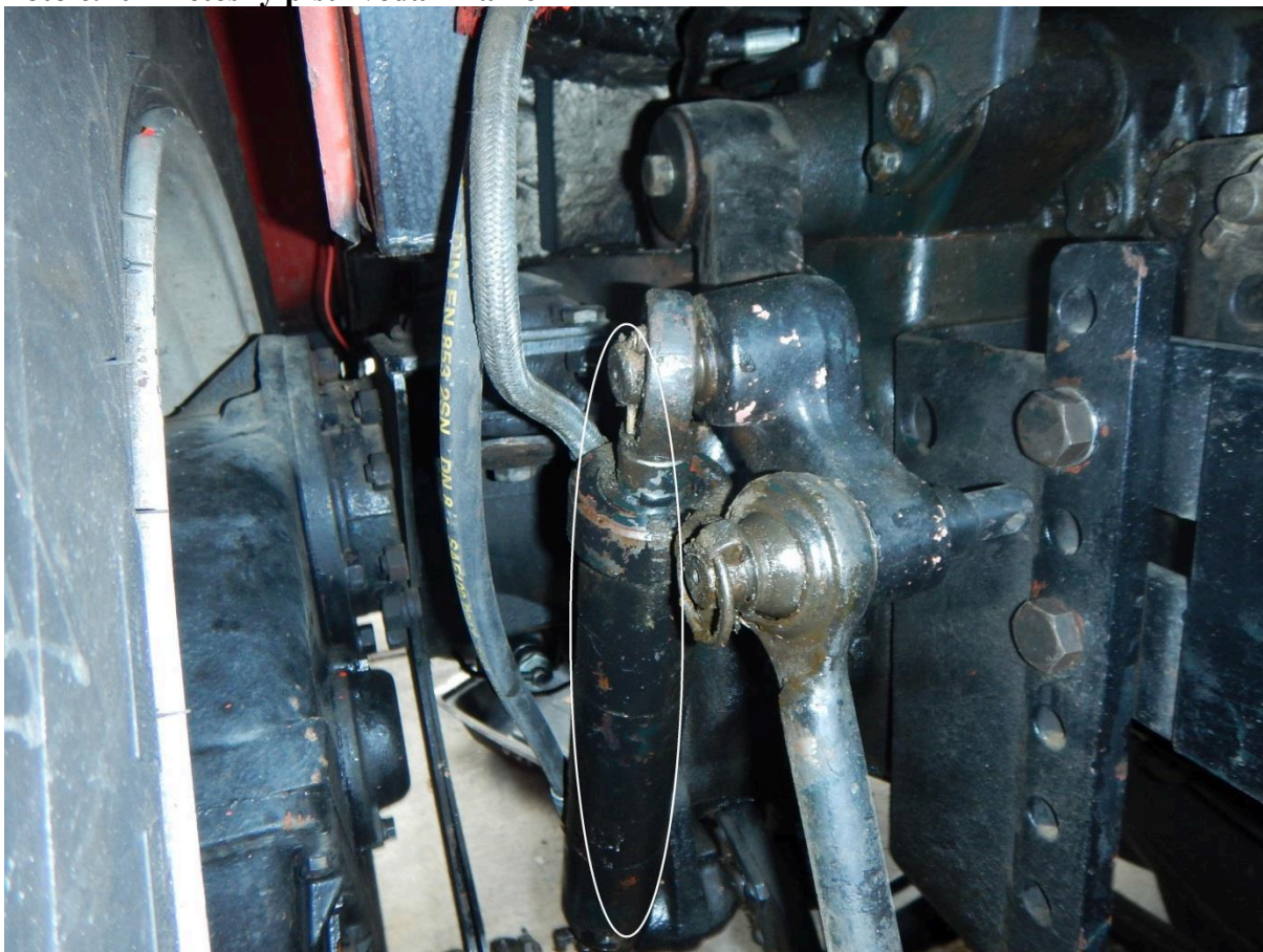
Foto č.20 – netěsný píst zvedání ramen
