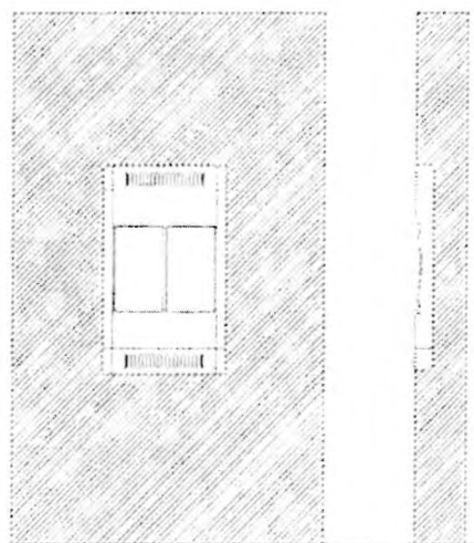
Instalace do niky, s větracími otvory nad a pod modulem
