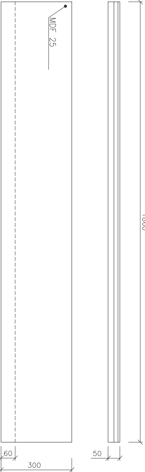
DETAIL TRUHLÁŘSKÉHO PRVKU M1:10
