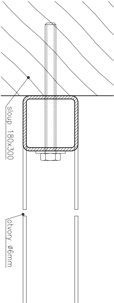
DETAIL KOTVENÍ ZÁMEČNICKÉ KONSTRUKCE M1:2
