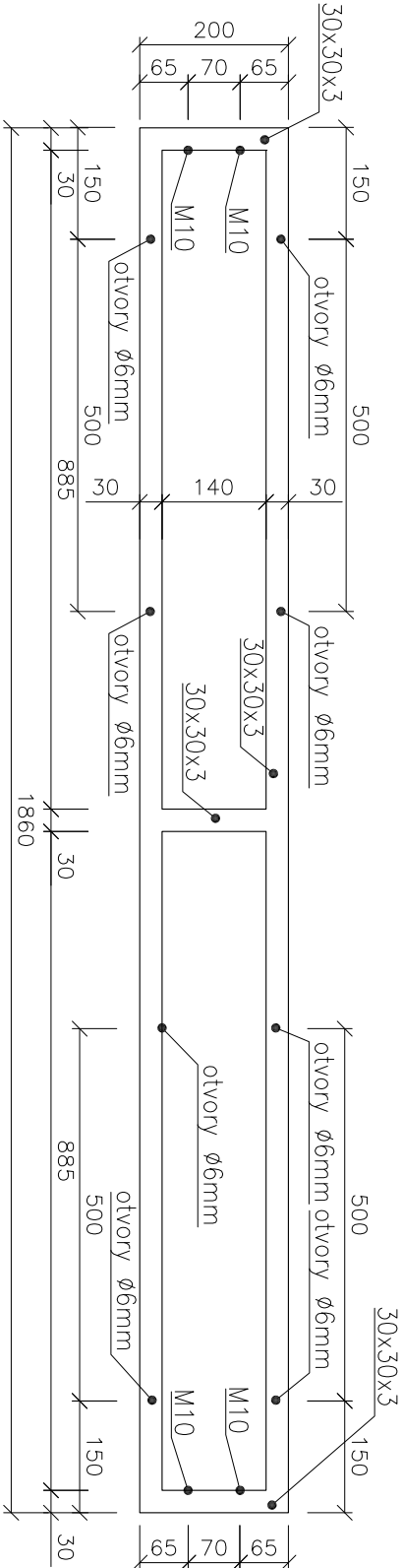
DETAIL ZÁMEČNICKÉ KONSTRUKCE M1:10
