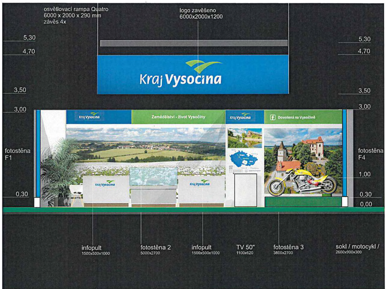
pohled čelní 1_50
