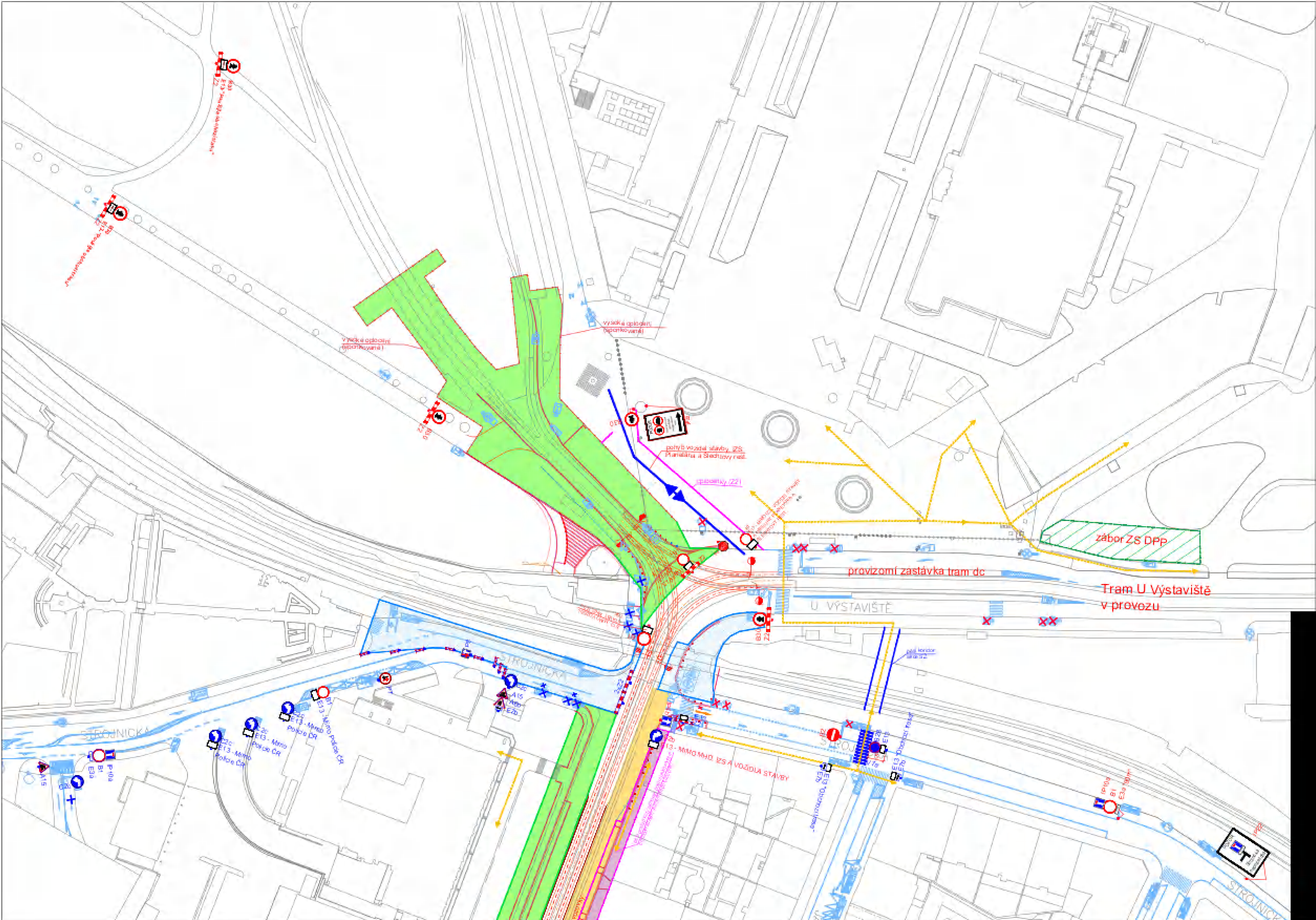
Situace - vjezd do Stromovky z Ovencecké M1:500
