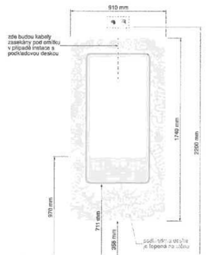
VARIANTA B dotažení zásuvek k panelu (doporučujeme nad panel)
