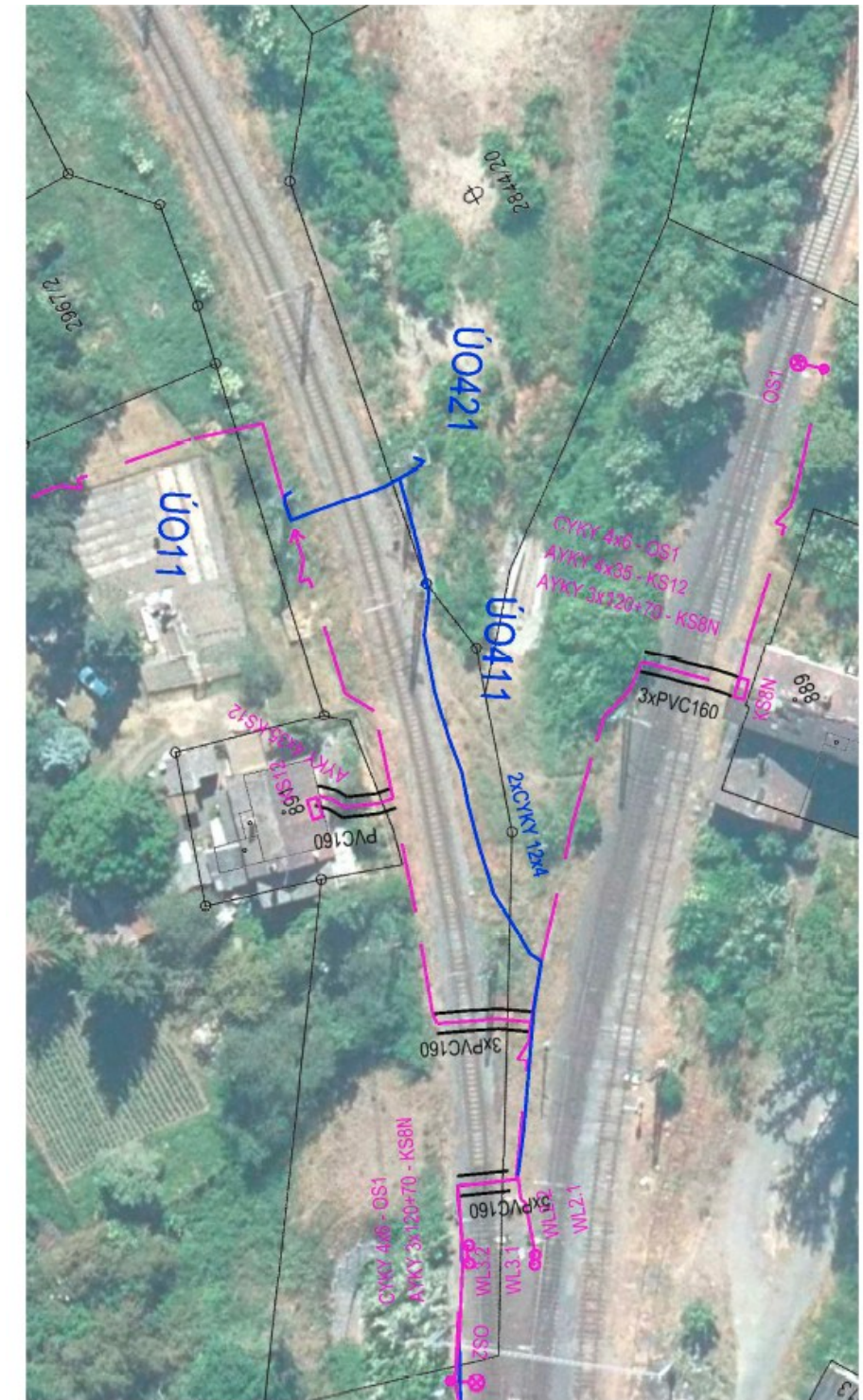
č. 2 – Zákres trakčního stožáru včetně kabelového vedení
