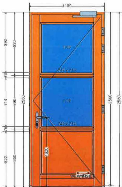
Vnitřní pohled
