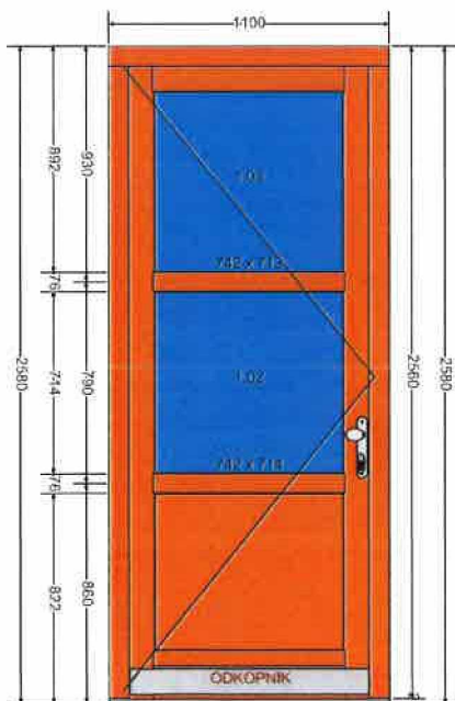
Vnitřní pohled
