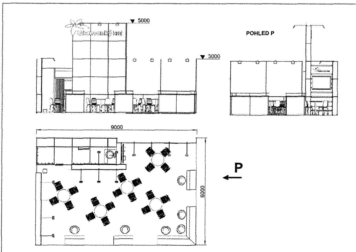
Základní pohledy s rozměry Stavotech 2016
