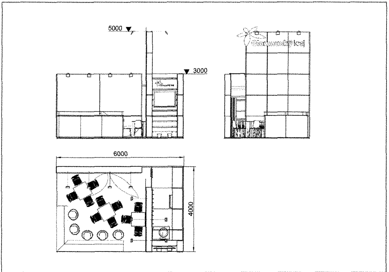
Základní pohledy s rozměry MSV 2016
