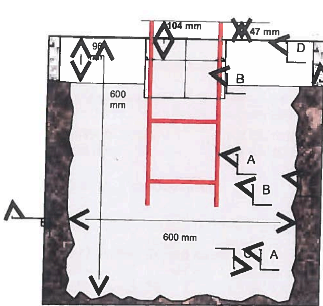
Varianta č. 4 (ovládací prvky ve výšce 1300 mm)
