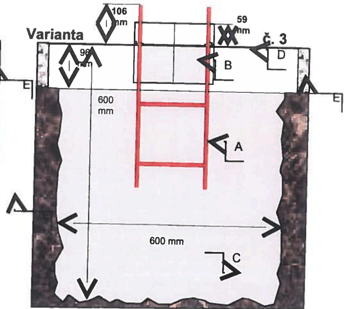
Varianta č. 3 (ovládací prvky ve výšce 1337 mm)
