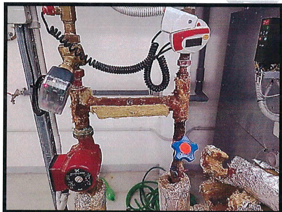
Staré potrubí:
