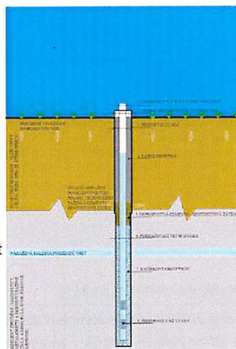
Obr. Řez vrtané studny 222/191 - 125mm mm
