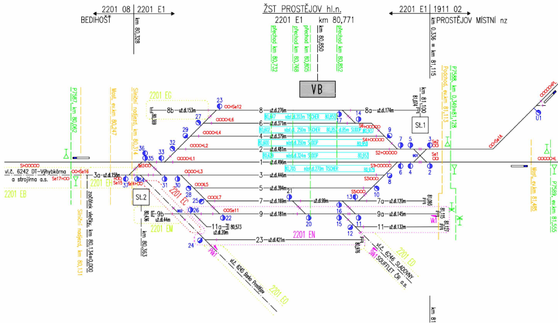
Situační plán
