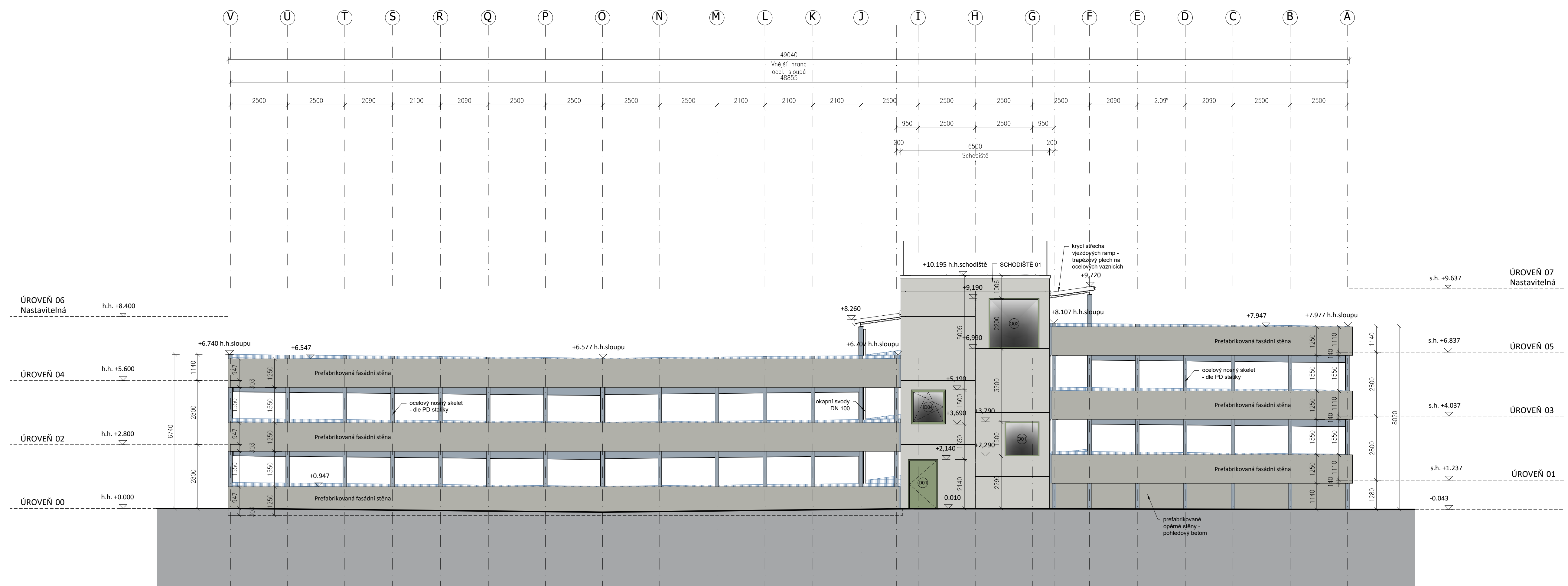
POHLED JIHOZÁPADNÍ
