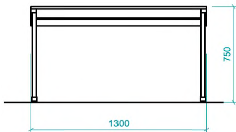
POHLED ČELNÍ:
