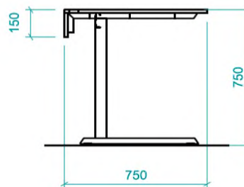
POHLED BOČNÍ:
