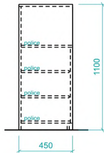
POHLED BOČNÍ:
