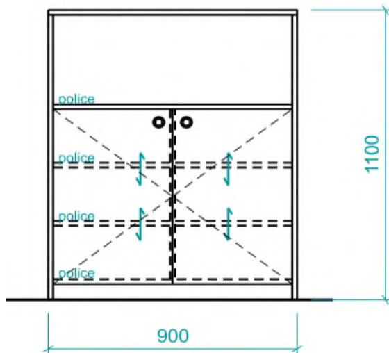
POHLED ČELNÍ:
