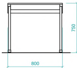
POHLED ČELNÍ:
