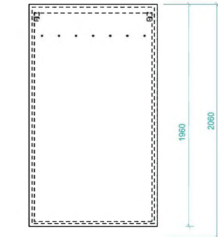
POHLED ČELNÍ:
