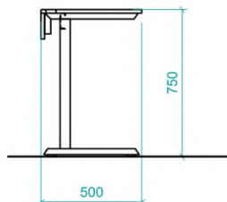
POHLED BOČNÍ:
