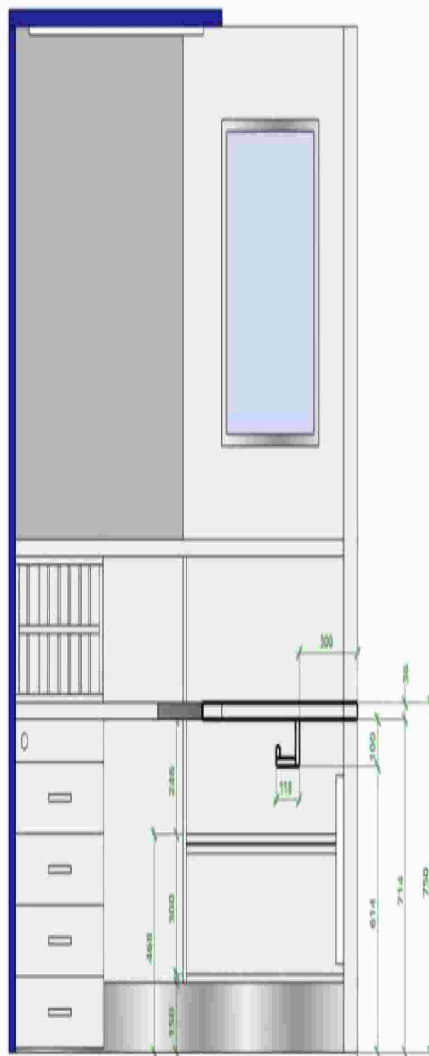
ŘEZ 02:
