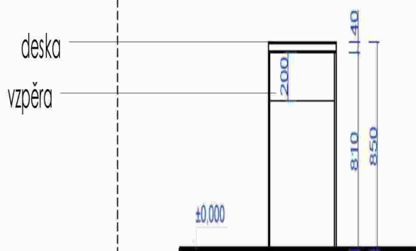
řez
