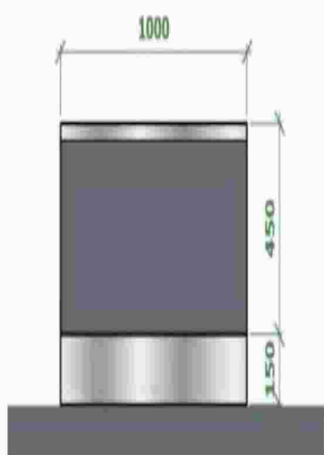
POHLED:
