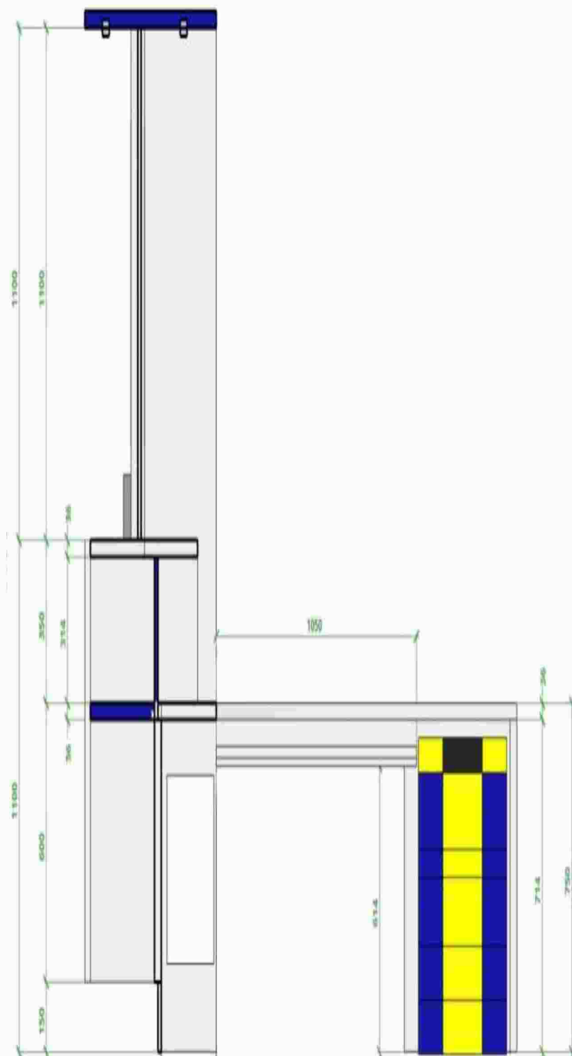
ŘEZ 01:
