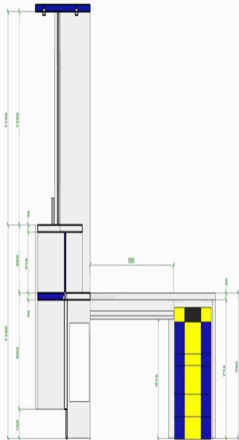
ŘEZ 01:
