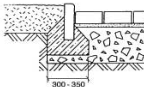
Vzor uložení obrubníků a zámkové dlažby:
