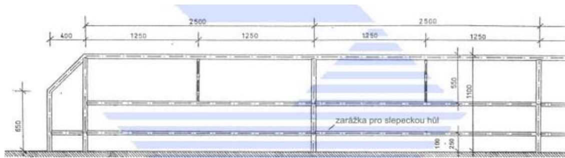
Obrázek 5 – Schéma silničního (dopravně bezpečnostního) zábradlí s výplňovým prutem a zarážkou pro slepeckou hůl
