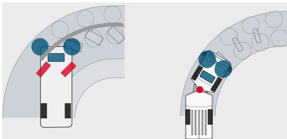
Vozidlo s řízením na přední nápravě | BUCHER CityCat V20 s kloubovým řízením
