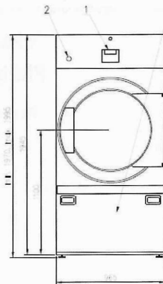
ČELM POHLED
