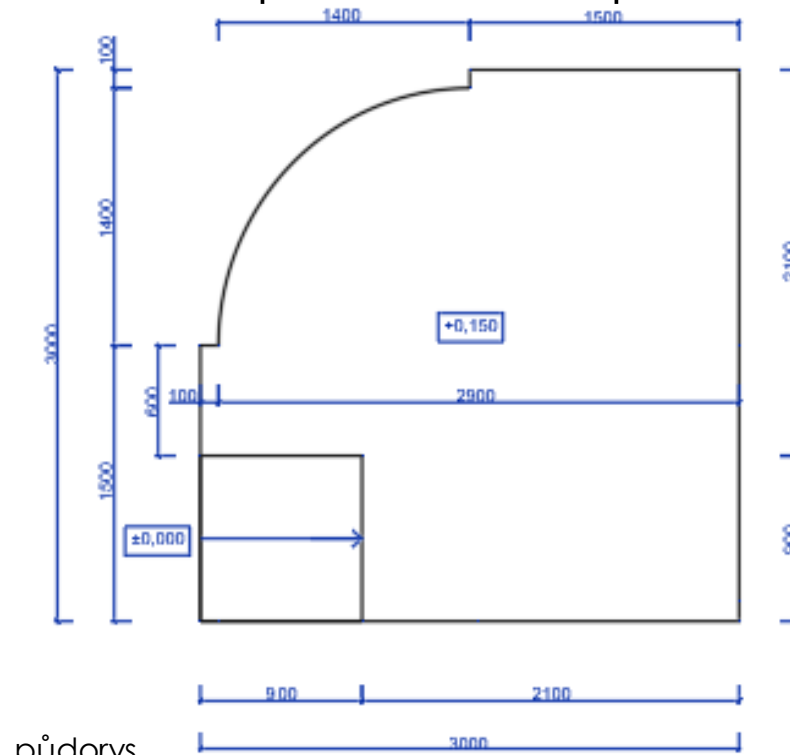
půdorys
