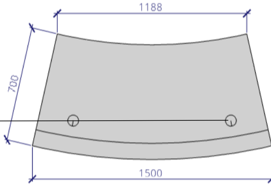
půdorys
