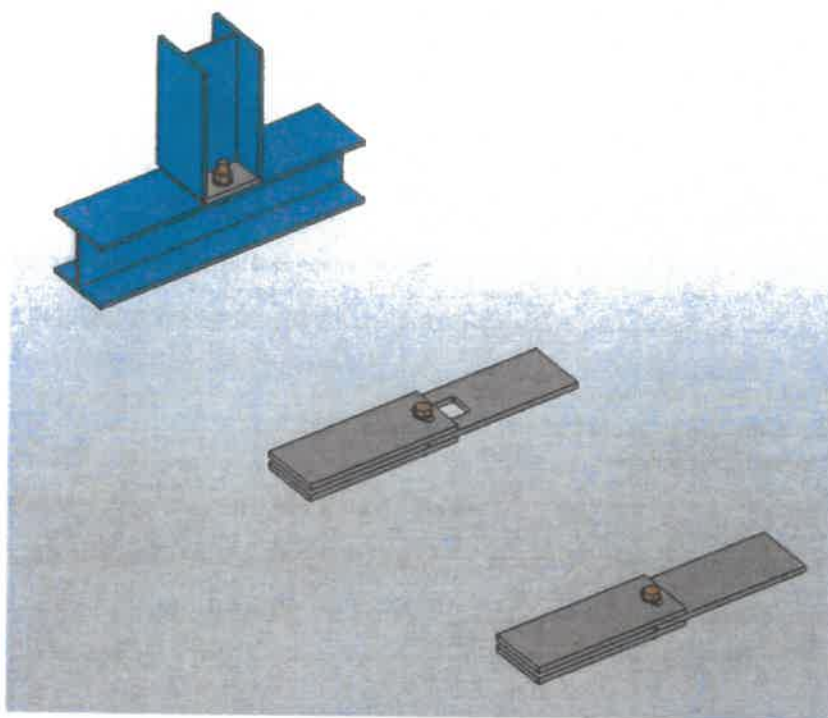
Obrázek 1 – 3D pohled na 3 řešené varianty
