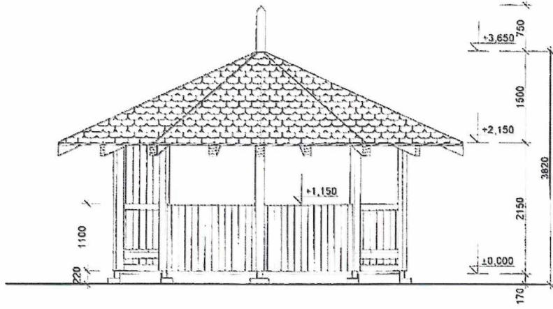
POHLED 1:50
