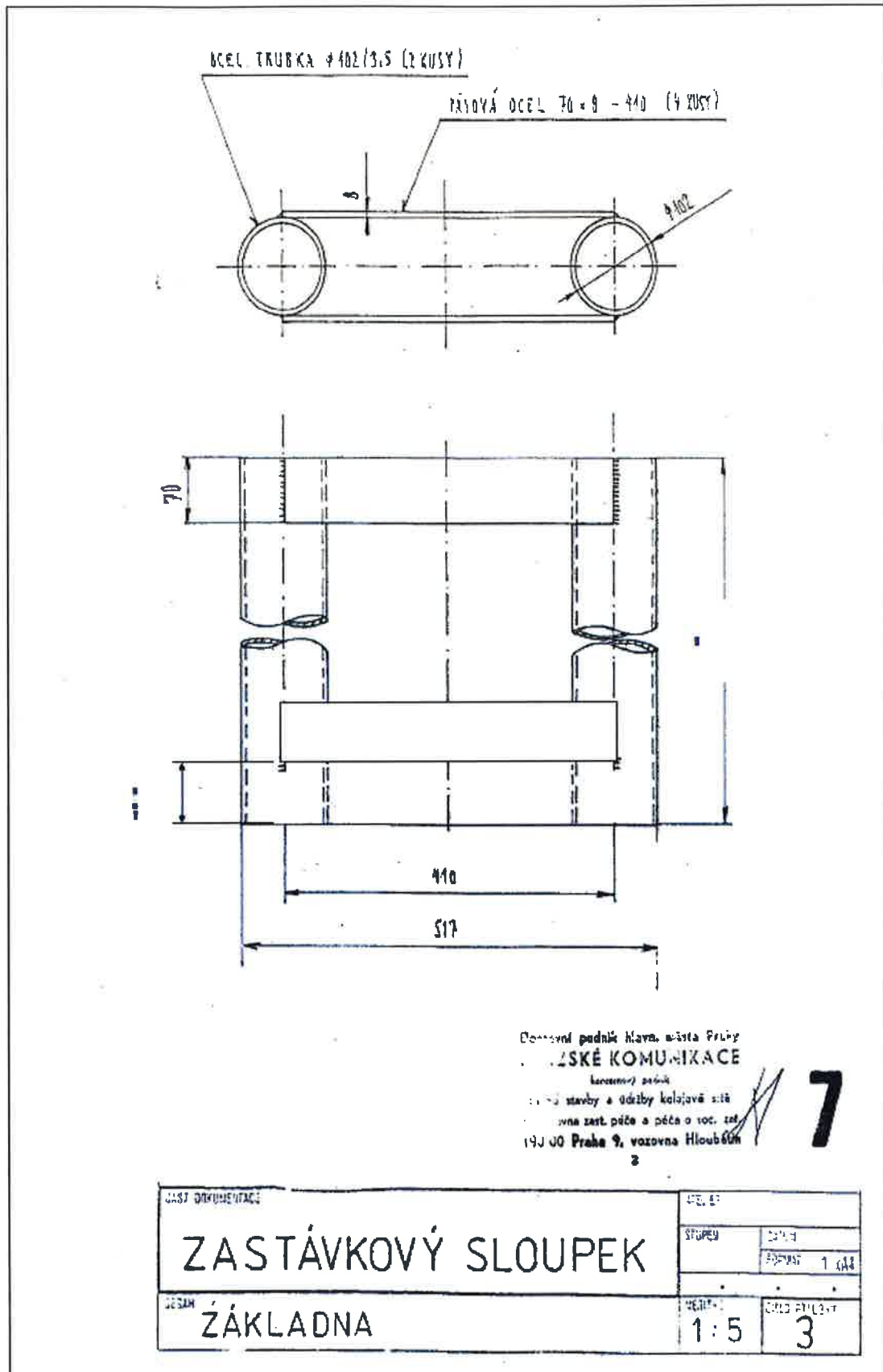
Obrázek 2: Schéma základny označnicku
