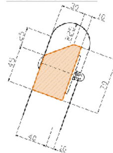
DET. A ZKOSEŇÍ HORNÍ LATĚ
