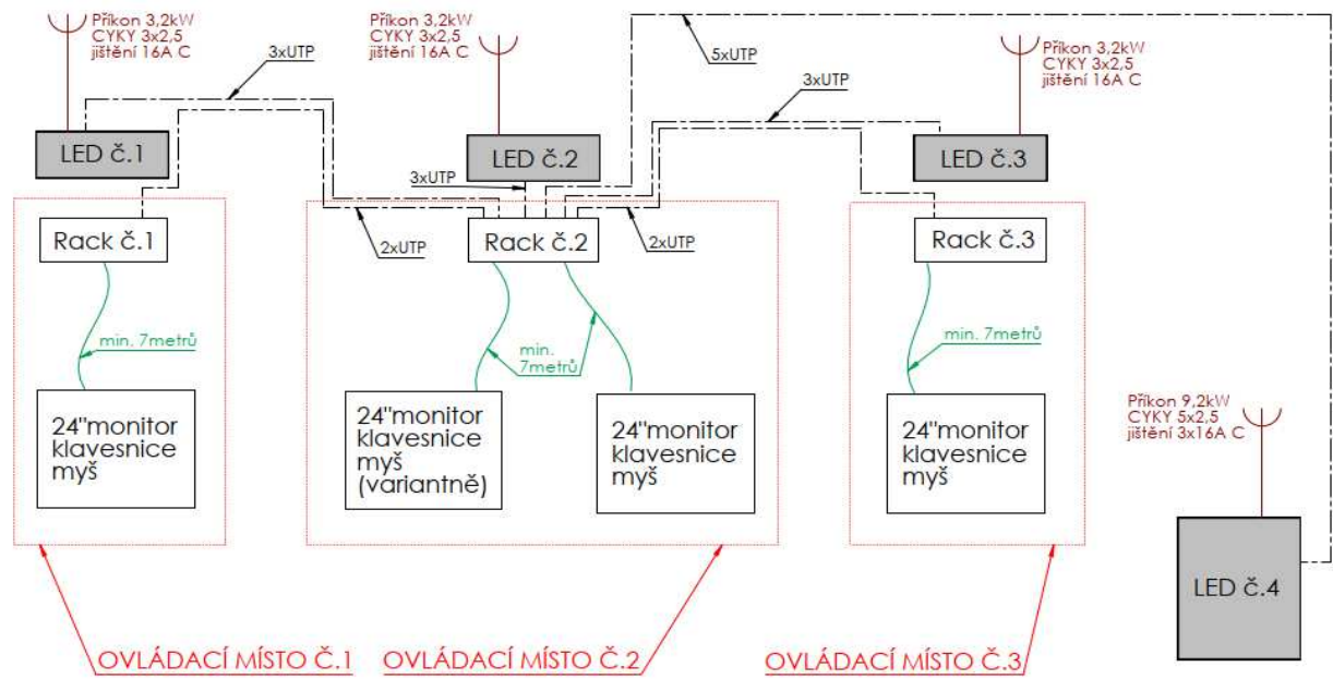
Schéma zapojení ATLAS II
