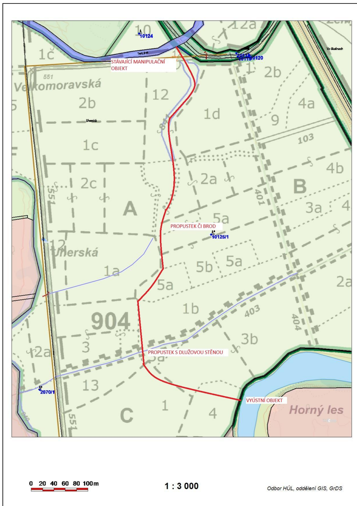
Příloha č. 3. Podrobná situace s vyznačením navrhovaných opatření
