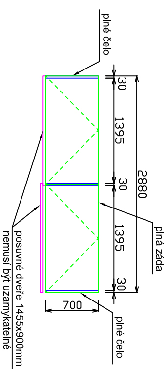
ZÁSUVKOVÁ SKŘIŇ - m.č. 404
