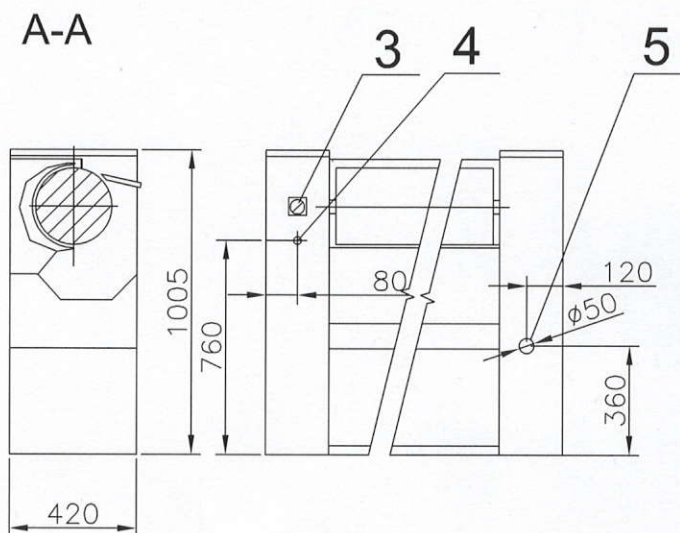
BOČNÍ POHLED
