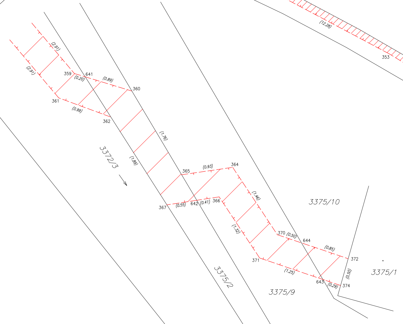
Detail:C
