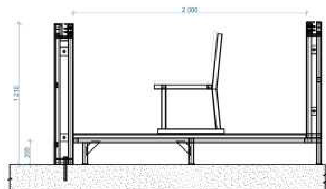
ŘEZ STŘIDAČKOU M 1:20
