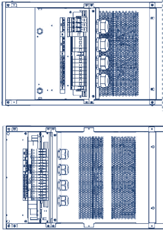
Zadní panel svorkovnice Force 10–20 kVA
